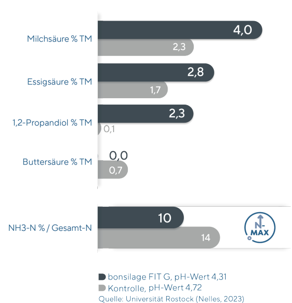
Verbesserte Gär säuren- und NH 3 -N-Gehalte am Siliertag 90 – Grassilage mit ca. 30 % TM
