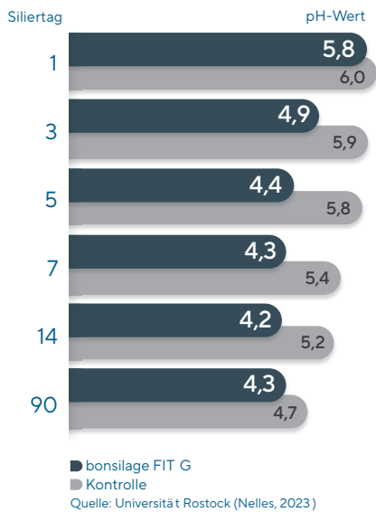
Schnellerer pH-Wert Abfall über alle Siliertage – Grassilage mit ca. 30 % TM
